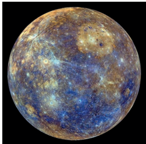
La teoria del camp gravitatori va descriure bé l'anomalia de l'òrbita de Mercuri tot i que la causa no va ser explicada fins a la teoria de la relativitat general d'Einstein.
