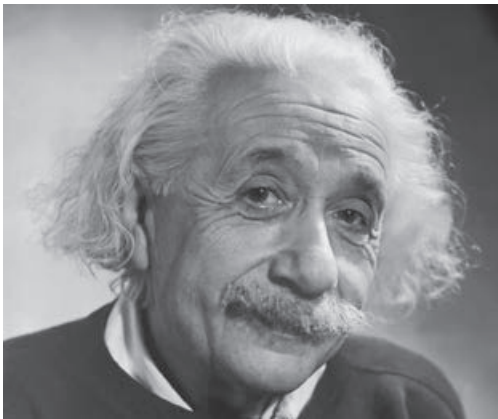
La teoria de la relativitat general d'Albert Einstein (1879-1955) porta la matematització del món fins als aspectes més extrems tot fent de l'espai el principal protagonista còsmic.
