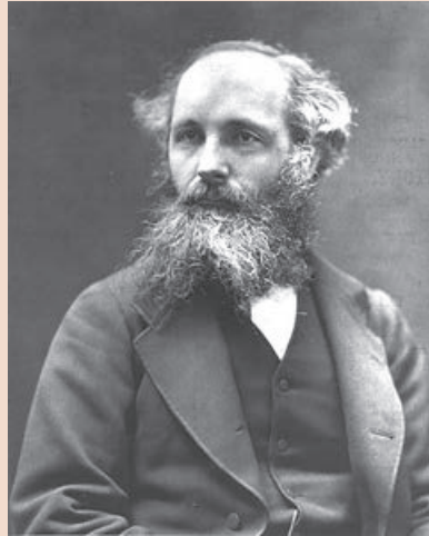
Les equacions de Maxwell que regeixen el camp magnètic i el camp elèctric van ser comprovades empíricament per Hertz i van ser aplicades per Marconi amb l'invent de la ràdio.
